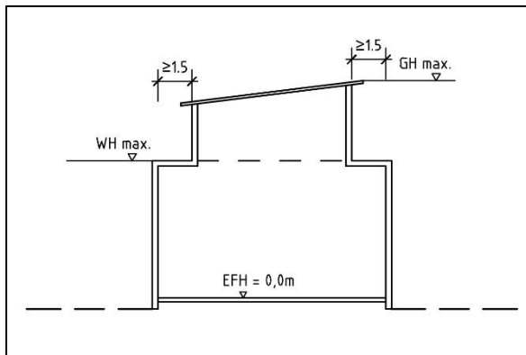
Abbildung 10: Schemaschnitt Staffelgeschoss; Zink Ingenieure
